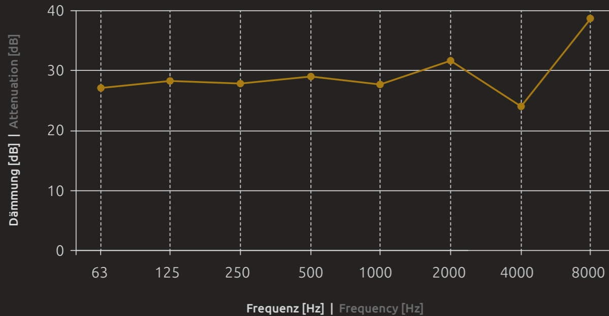
DÄMMKURVE (Mittelwert der Schalldämmung) ATTENUATION CURVE (Average value of sound attenuation)
